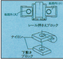
平面図
